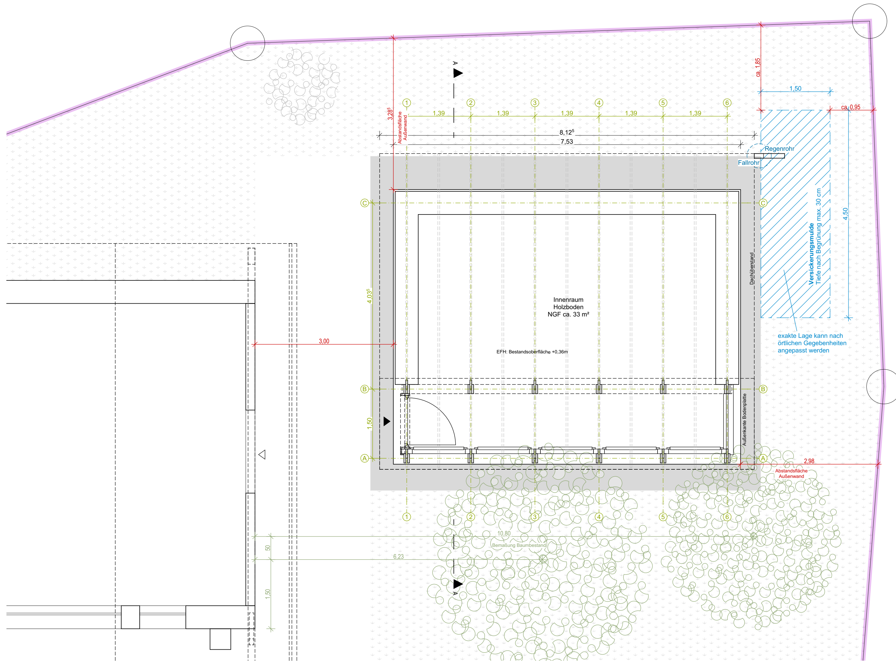
Planzeichnung für Sickermulde
