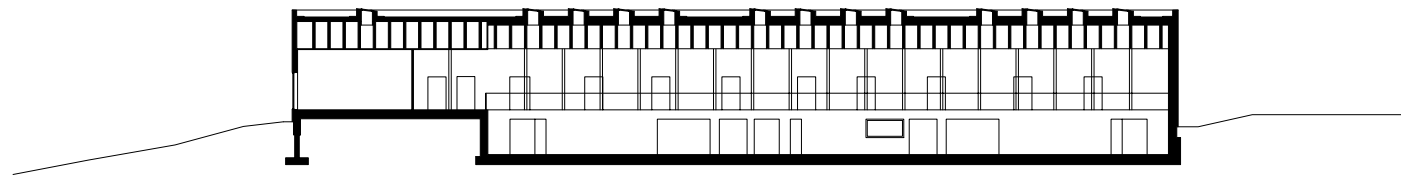
Schnitt A
