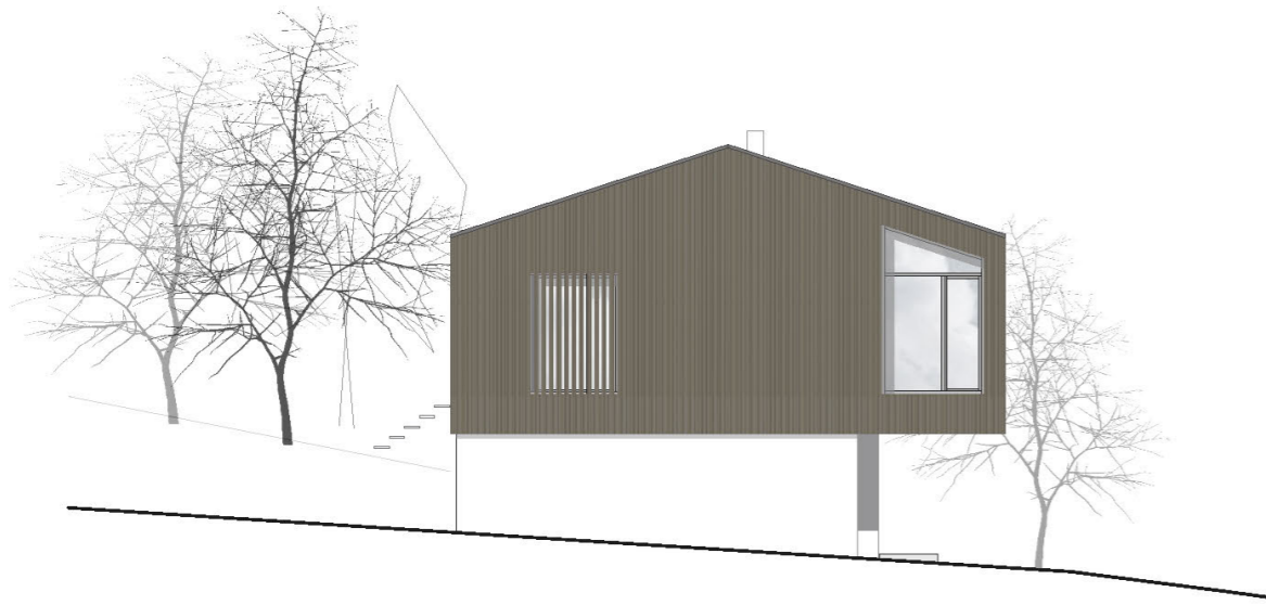
ANSICHT NORD
