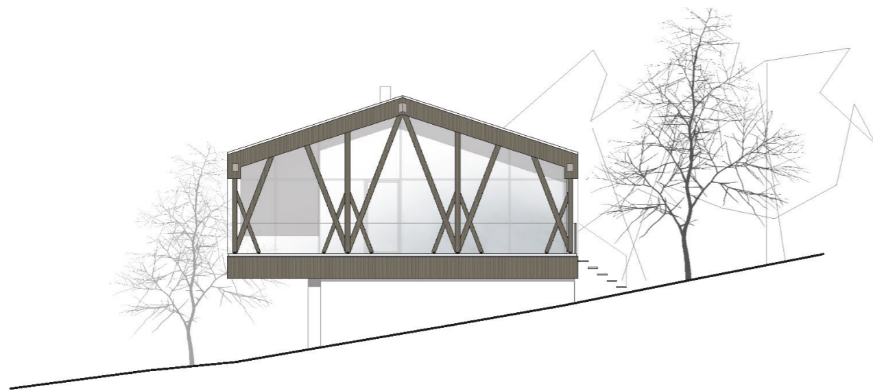
ANSICHT SÜD
