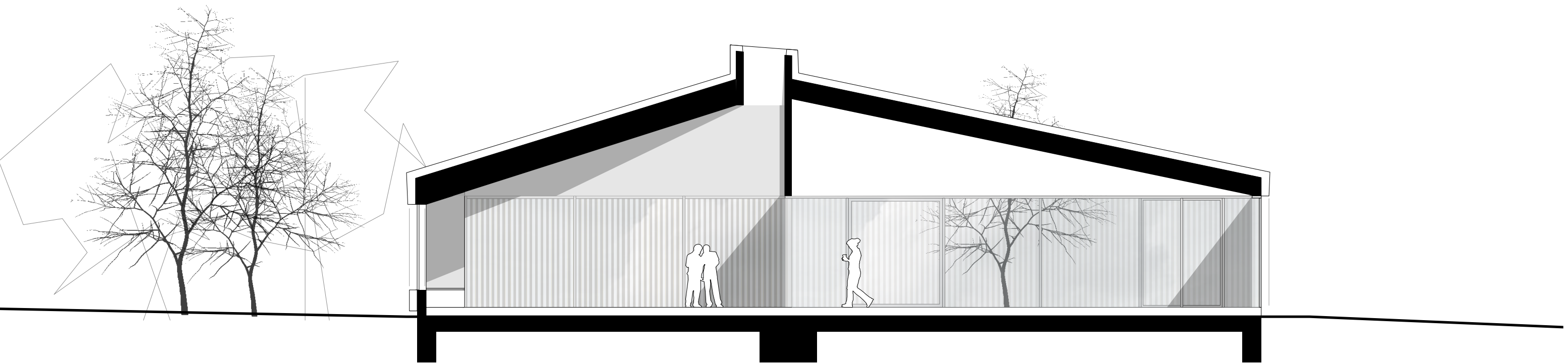
Schnitt B-B
