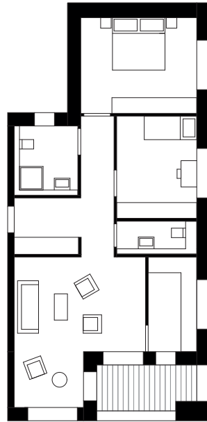
Lameygarten, Mannheim - Wohneinheit - 1:50
